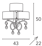
Elena 3023/A3L 3 x max 60W E14 230V
