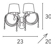
Erica 3021/A2L 2 x max 60W E14 230V
