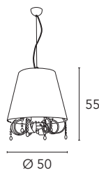
Erica 3021/S4L 4 x max 60W E14 230V
